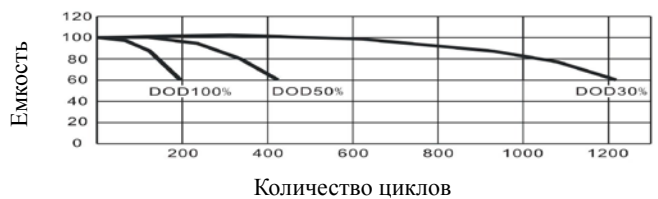
Зависимость срока службы от глубины разряда
